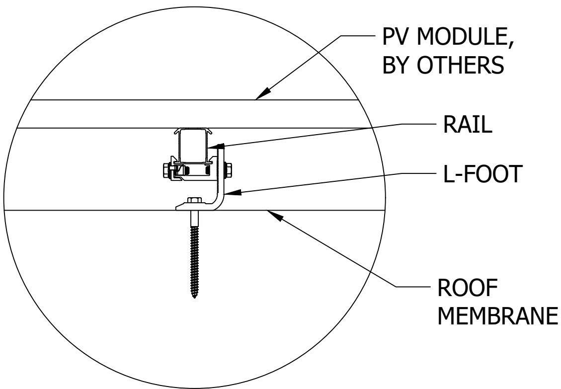
H GF-1 DETAIL SIDE Scale: 3"=1'-0"
