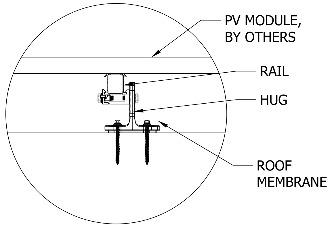
H HUG DETAIL SIDE Scale: 3"=1'-0"
